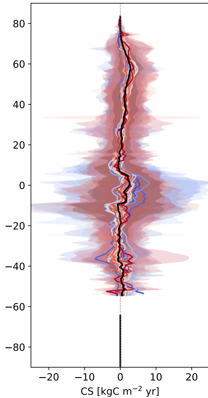
b) TRENDY
