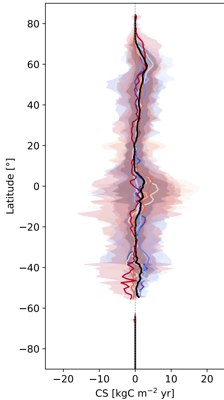
a) CMIP6
